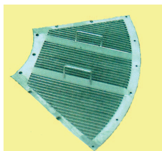
Telas com bordas de PU para Peneira Kambalda
